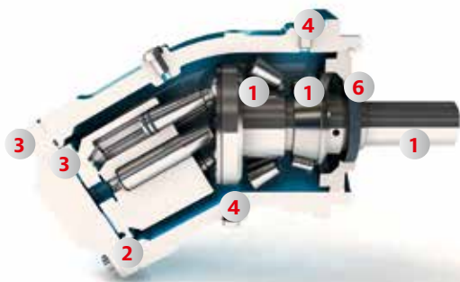
Bomba Hidráulica
